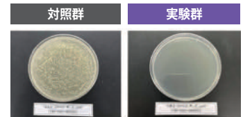
E.coli(大腸菌)
